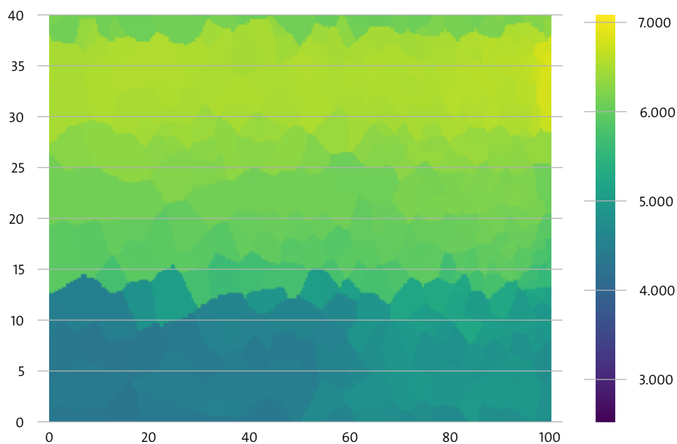
Abbildung 14: Vom ML-Modell vorhergesagte Anzahl an Fahrradleiher für synthetische Datenpunkte, bei denen ausgehend von einem spezifischen Datenpunkt die Attributwerte von Temperatur und Luftfeuchtigkeit variiert wurden.
