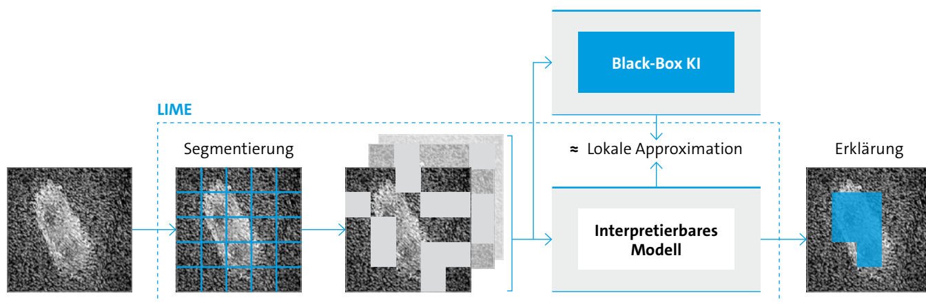
Abbildung 5: LIME am Beispiel eines Textilfehlers. Relevante Bereiche für die Klasse Klebereste sind in der Erklärung farblich markiert.
