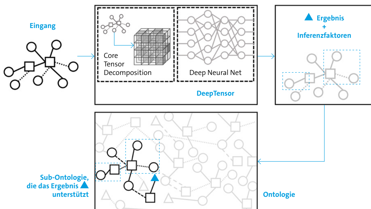
Abbildung 7: Erklärung durch Kombination von DeepTensor und Ontologien
