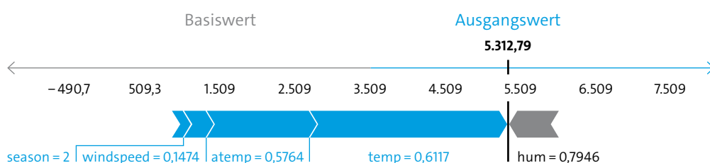
Abbildung 13: Erklärung einer einzelnen Modellvorhersage mithilfe des SHAP Verfahrens. Analog zu LIME wird der Effekt einzelner Attributwerte auf den Vorhersagewert des Modells für einen gegebenen Datenpunkt visualisiert. Wirkliche und gefühlte Temperatur, Windgeschwindigkeit und Jahreszeit haben einen positiven Einfluss, die Luftfeuchtigkeit hat einen negativen Einfluss auf den Vorhersagewert. Unten: Werte der einzelnen Attribute für den gegebenen Datenpunkt.
