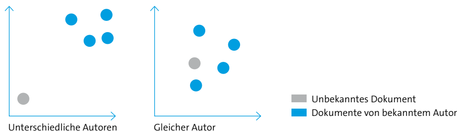
Abbildung 15: Die Stilvektoren zweier AV-Fälle, visualisiert mithilfe der Dimensionsreduzierungstechnik t-SNE [7]. In beiden Fällen bilden die Vektoren der Dokumente der jeweiligen bekannten Autoren (blau) eine dichte Gruppierung. Das unbekannte Dokument (grau) des linken Falls wurde von einem anderen Autor verfasst und liegt entsprechend distanziert zu der Gruppierung des anderen Autors. Im rechten Fall dagegen handelt es sich um ein Dokument des bekannten Autors und mischt sich dementsprechend unter die Gruppierung.
