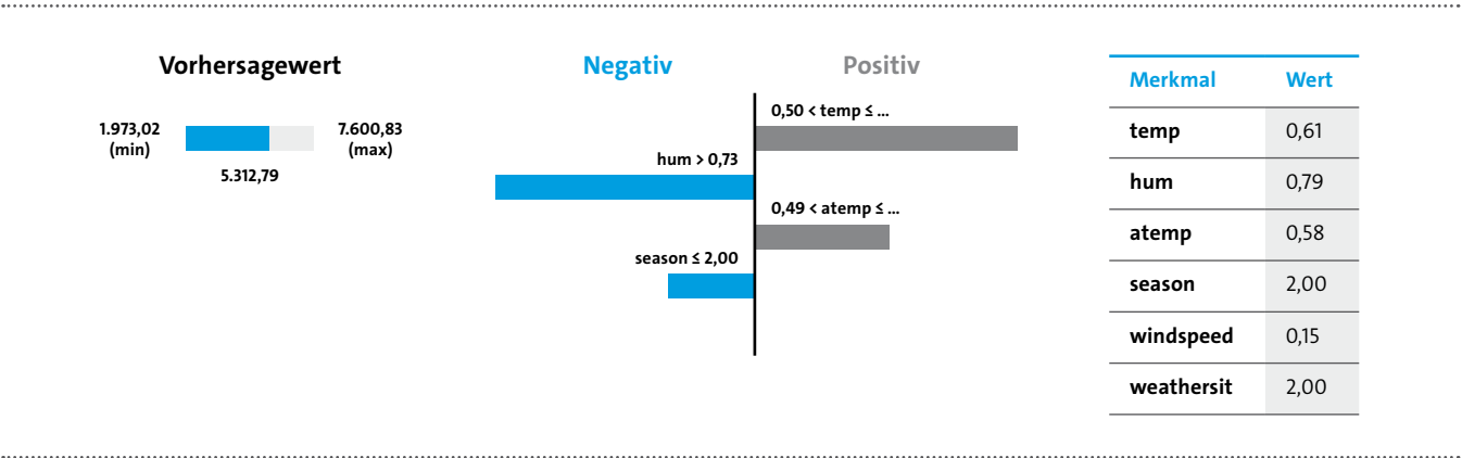
Abbildung 12: Erklärung einer einzelnen Modellvorhersage mithilfe des LIME Verfahrens. Links: Vorhersagewert des Modells für die gegebenen Eingabewerte, mit Angabe des Minimum- und Maximumwertes der Modellvorhersagen. Mitte: Einfluss einzelner Attributwerte auf den Ausgabewert. Wirkliche und gefühlte Temperatur wirken sich positiv auf den Vorhersagewert aus, Luftfeuchtigkeit und Jahreszeit negativ. Rechts: Eingabewerte aller betrachteten Attribute für die gegebene Modellvorhersage.
