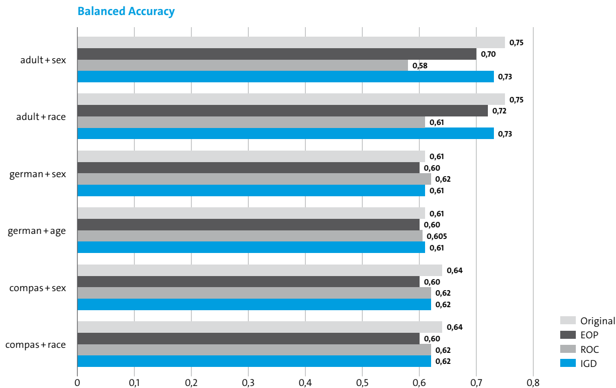
Abbildung 24: Ausgewogene Genauigkeit der verschiedenen Verfahren zur Bias-Reduzierung
