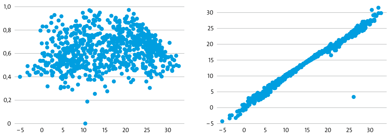
Abbildung 10: Links: Abhängigkeit der Luftfeuchtigkeit von der Temperatur im Beispiel-Datensatz. Rechts: Abhängigkeit der gefühlten Temperatur von der wirklichen Temperatur.
