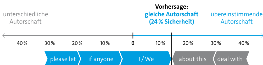
Abbildung 16: Der Entscheidungsprozess für ein AV-Fall verdeutlicht als Zusammenspiel aus mehreren Merkmalen. Merkmale beeinflussen die finale Entscheidung ausgehend vom Schwellenwert \theta entweder in Richtung übereinstimmender Autorschaft (blau, nach rechts) oder unterschiedliche Autorschaft (grau, nach links). Sie sind dabei abhängig ihrer Relevanz skaliert, sodass relevante Merkmale mehr zur Entscheidung beitragen und visuell hervorgehoben sind.
