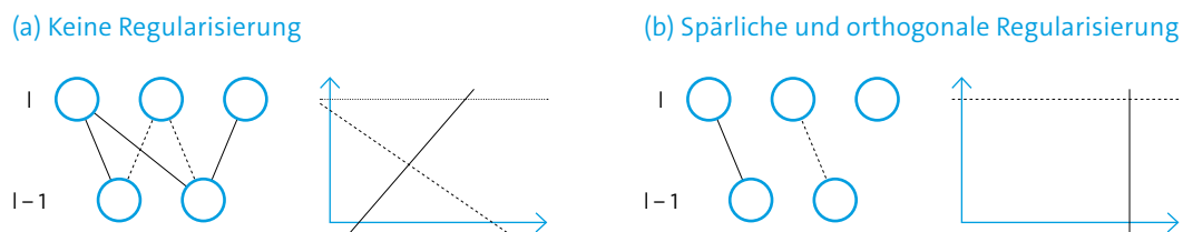
Abbildung 26: Auswirkung der Kombination aus spärlicher und orthogonaler Regularisierung auf die Gewichtsvektoren eines MLP. In jeder Teilabbildung ist links ein MLP und rechts die Entscheidungsgrenzen der Neuronen der oberen Schicht dargestellt.
