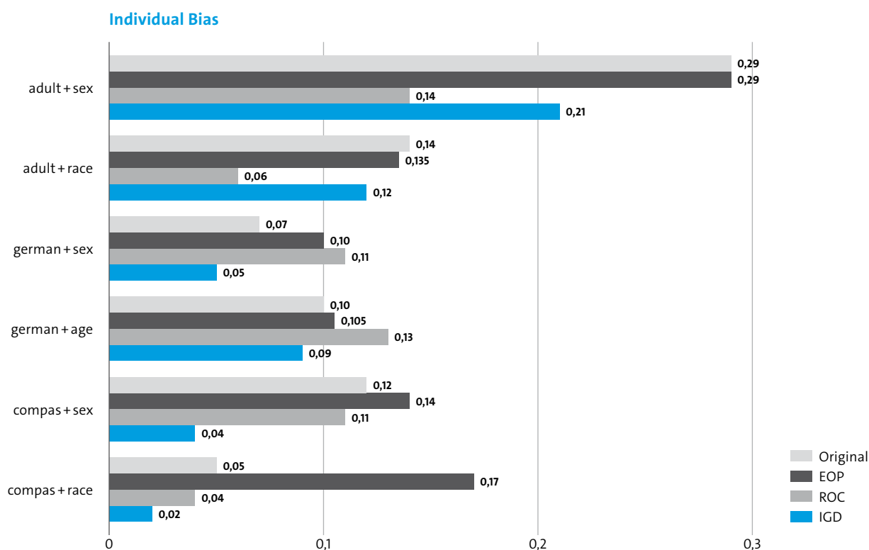
Abbildung 23: Individueller Bias Korrektur mit verschiedenen Attributen. Die Datensätze UCIAdult (adult), UCI Statlog German Credit (german) und ProPublica COMPAS (compas) wurden dazu herangezogen und die jeweiligen Attribute (sex, race und age) überprüft
