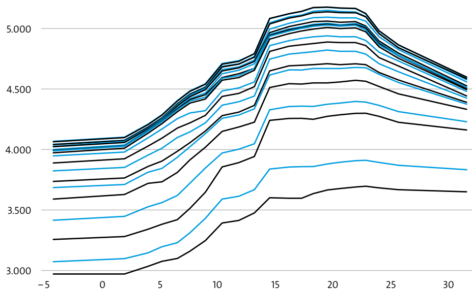
Abbildung 9: Partielle Abhängigkeit der Anzahl der Fahrradleiher von der Temperatur, dargestellt für verschiedene Werte der Luftfeuchtigkeit (je höher die Luftfeuchtigkeit, desto geringer die Anzahl der Fahrradleiher für eine gegebene Temperatur).
