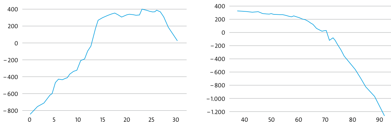
Abbildung 11: Links: Akkumulierter lokaler Effekt der Temperatur auf die Anzahl der Fahrradleiher. Rechts: Akkumulierter Effekt der Luftfeuchtigkeit.
