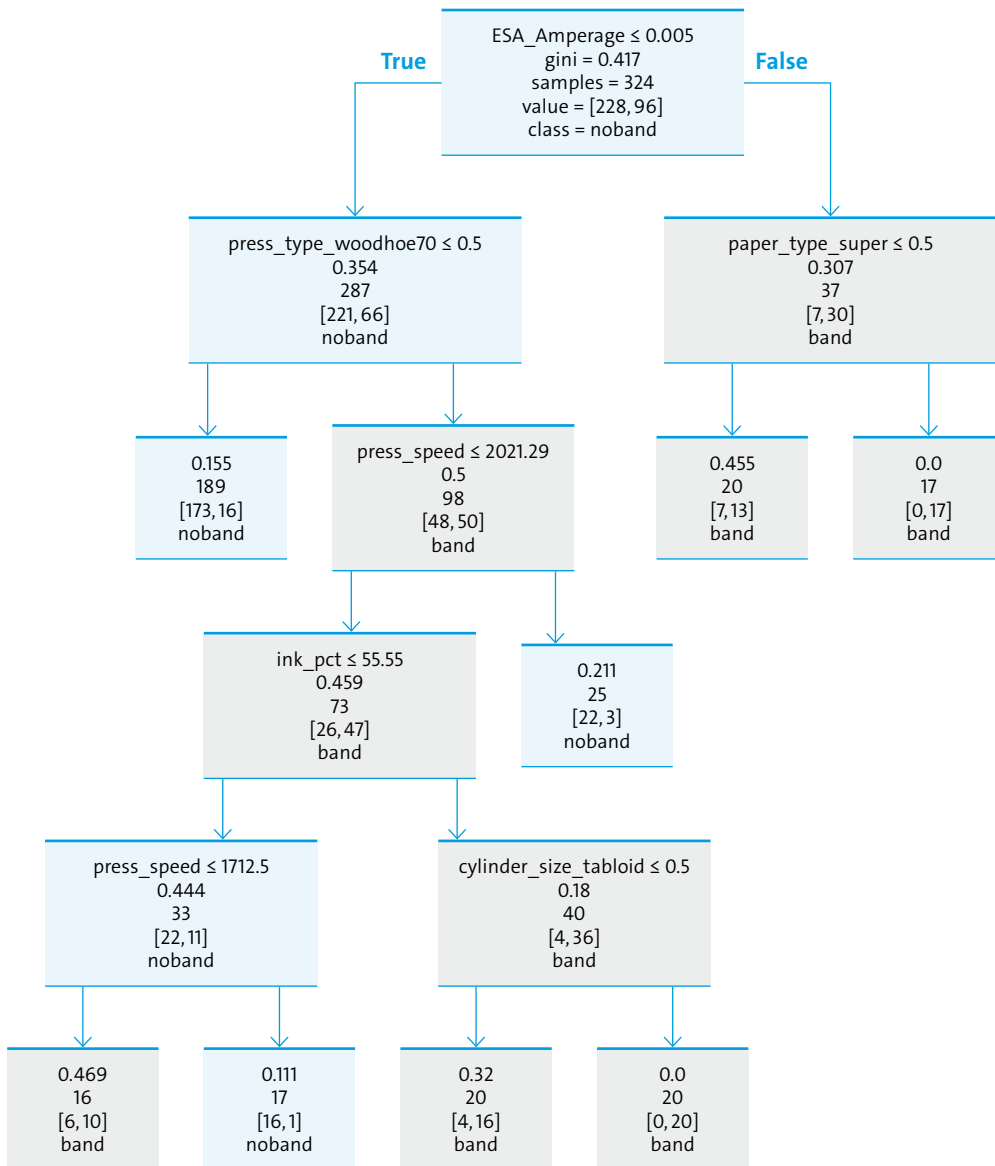
Abbildung 28: Entscheidungsbaum, extrahiert aus einem mittels SO-Regularisierung optimierten MLP. Der Baum hat eine APL von neun und einen Wiedergabetreuewert von 0,83.
