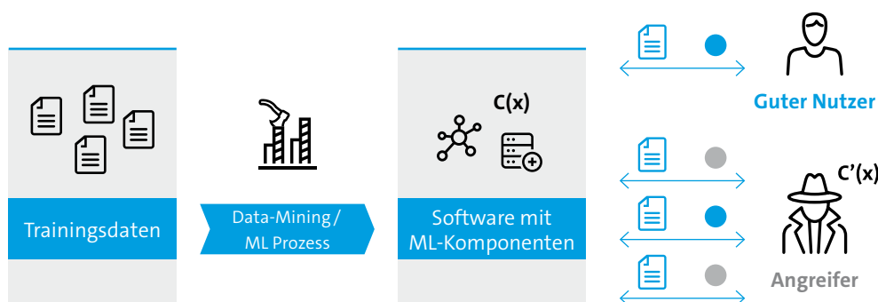
Abbildung 19: Prozess des feindlichen Angriffs auf KI: ein Angreifer, der sich mit dem Modell C(x) befasst, kann durch aktives Lernen zu seinem eigenen Verständnis des Modells als C'(x) gelangen. (Quelle: Sethi, Kantardzic, Ryu, 2017, »Security Theater«: On the Vulnerability of Classifiers to Exploratory Attacks)
