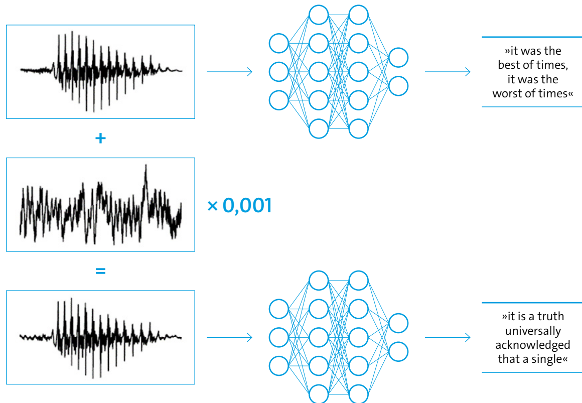
Abbildung 22: Feindliche Angriffe bei Audio Signalen in der automatischen Spracherkennung (Quelle: Carlini und Wagner 2018)
