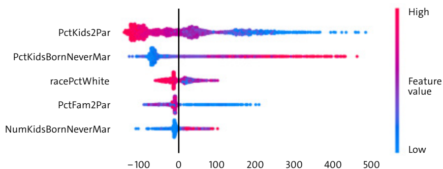
Abbildung 32: SHAP Value am Beispiel eines KI Systems zur Bewertung von Diabetes (Quelle: Eigene Darstellung)
