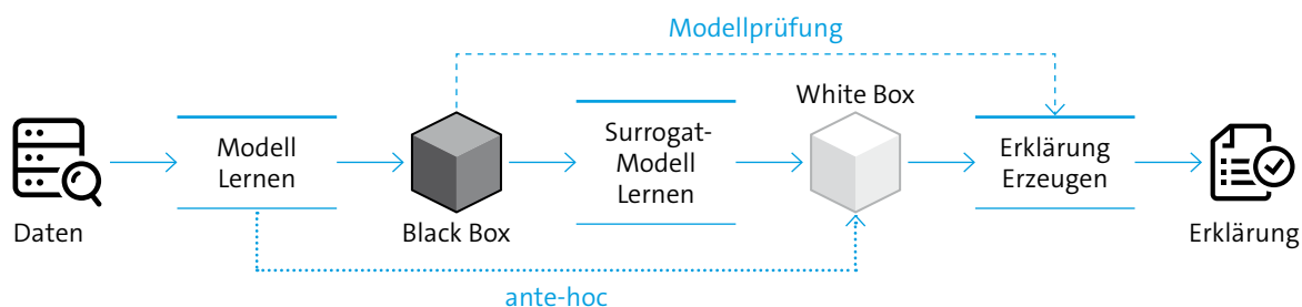
Abbildung 25: Von einem Black-Box-Modell zu einer Erklärung. Entweder durch direkte Erzeugung einer Erklärung aus dem Modell (gepunktete Linie, Modellprüfung) oder durch die post-hoc Extraktion eines interpretierbaren Stellvertretermodells (Surrogat), gefolgt von der Erzeugung von Erklärungen. Bei der ante-hoc Vorgehensweise (gestrichelte Linie) wird direkt ein interpretierbares ML-Modell erzeugt.
