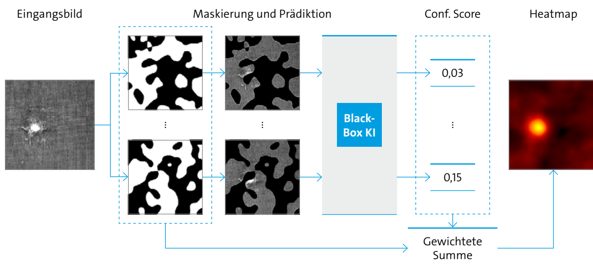
Abbildung 6: RISE Algorithmus am Beispiel eines Textilfehlers. In Anlehnung an [9]
