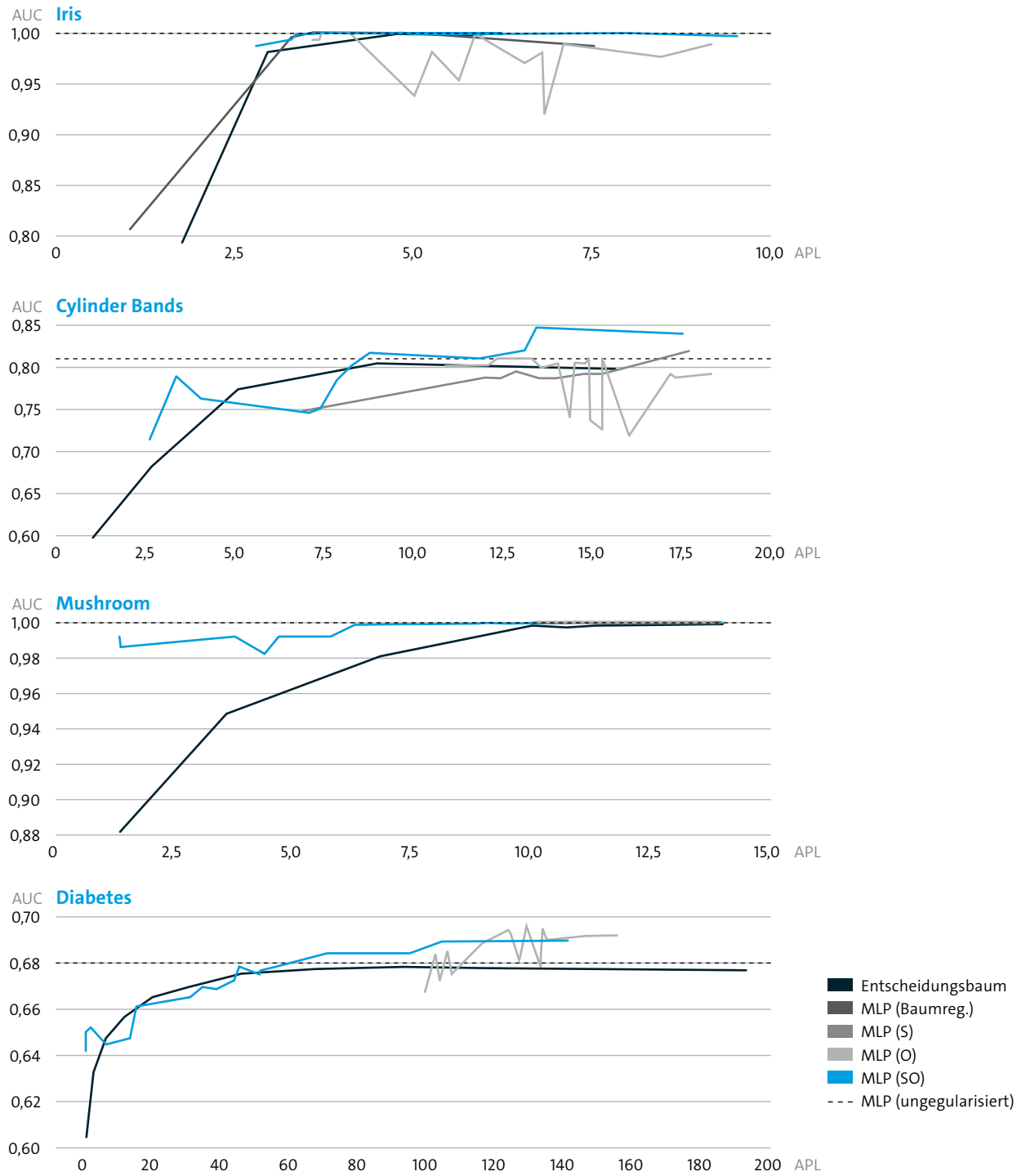
Abbildung 27: Entwicklung der Prognosegenauigkeit (AUC)
